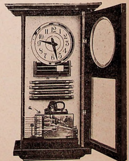
Fig. II. Centraalklok met schakelinrichting a.
