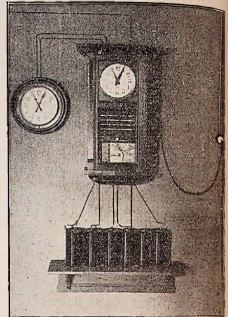
Fig. I. Complete draadloos bestuurd centraalklok met bijklok.
